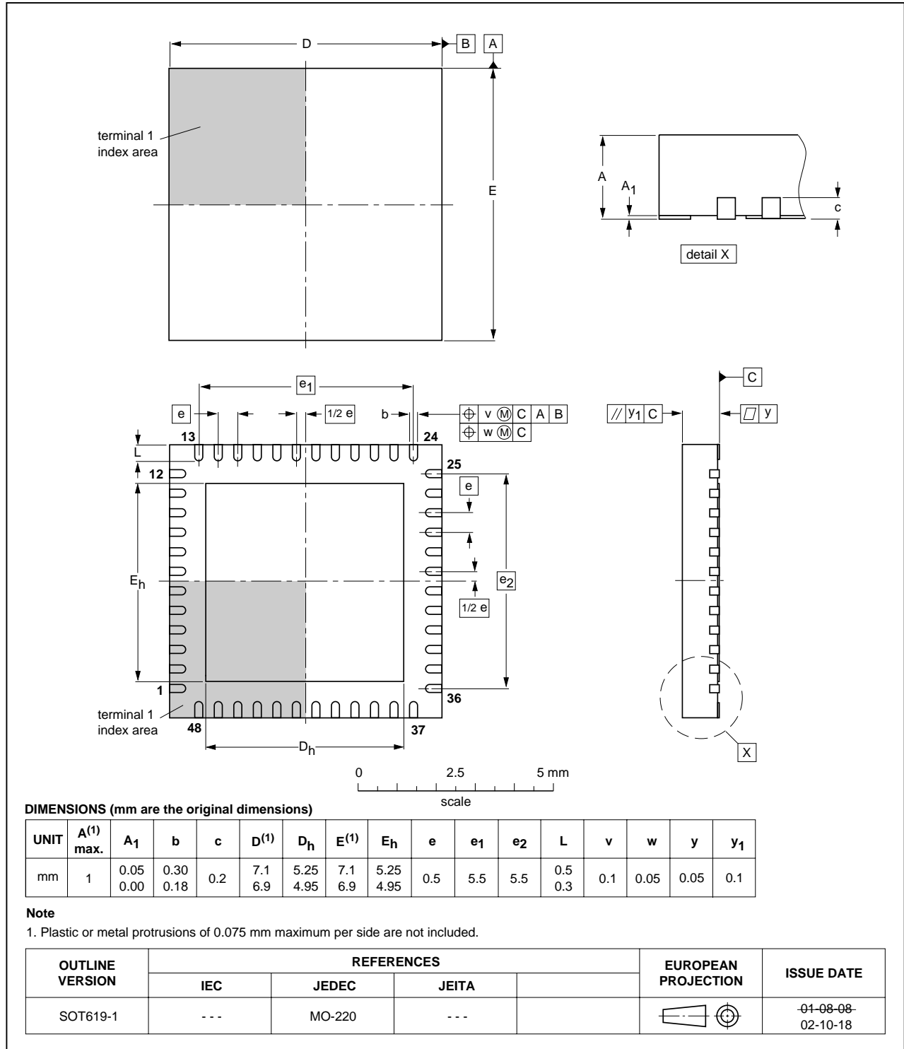
Fig 8. SOT619-1 (HVQFN48).
