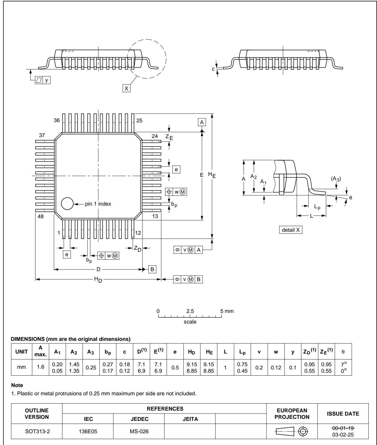
Fig 7. SOT313-2 (LQFP48).
